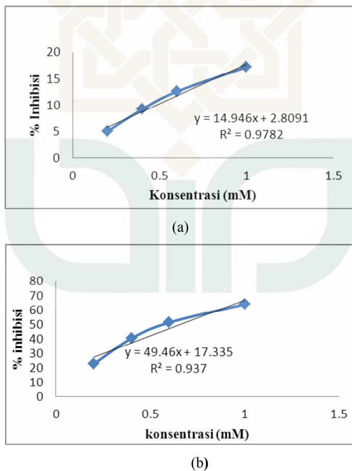
Gambar 6. Kurva konsentrasi terhadap % inhibisi dari vanilin (a); dan senyawa hasil sintesis (1,4-bis [(2-hidroksi-3-metoksi-5-metanal-fenil)-metil] piperazin) (b)
