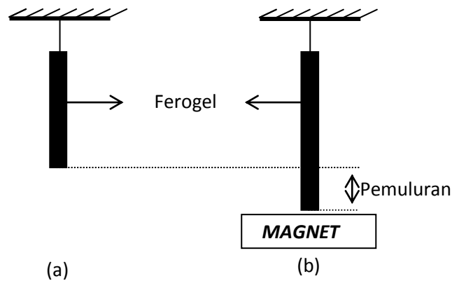
Gambar 4. Set alat eksperimen karakterisasi pemuluran ferrogel: (a) tanpa medan magnet; (b) dengan medan magnet
