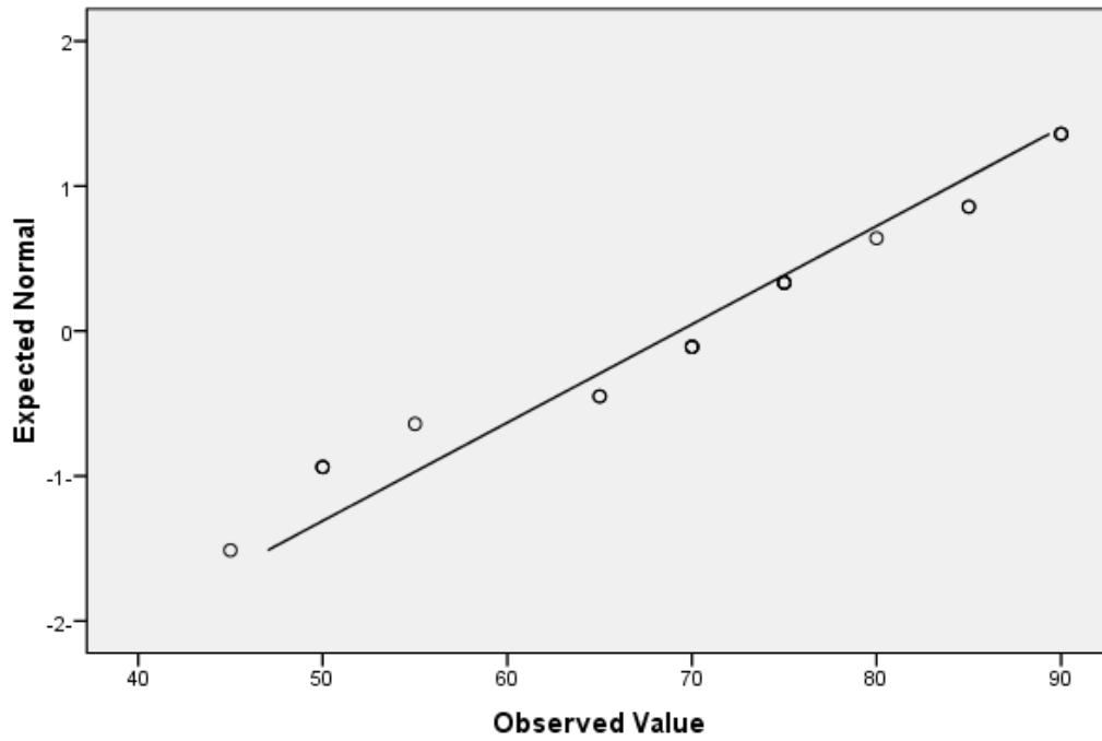
Normal Q-Q Plot of istima_kontrol
