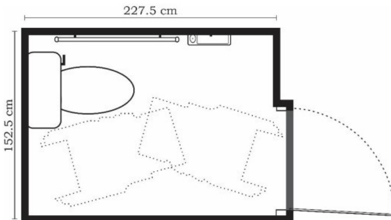
Dimensi minimal ruang dalam toilet penyandang disabilitas
