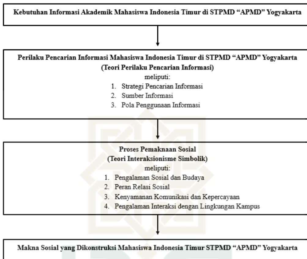
Gambar 1 Kerangka berpikir
