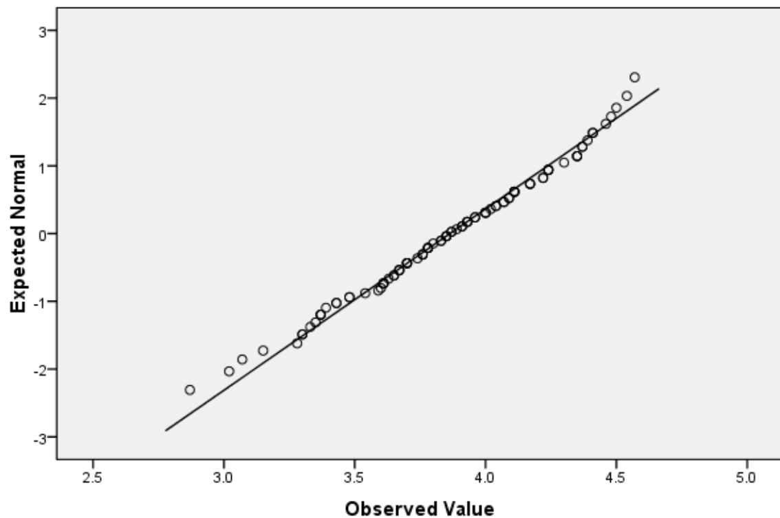
Normal Q-Q Plot of pembinaan keagamaan
